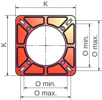
РЕКОМЕНДУЕМАЯ АМБРАЗУРА КОТЛА
